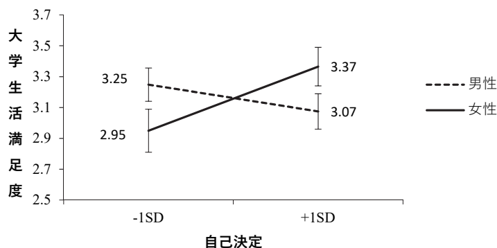
Figure 1. 自己決定と性別の交互作用における単純傾斜検定結果
