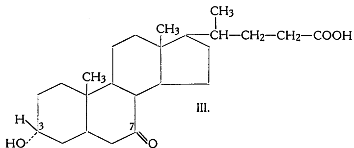
3-Oxy-7-ketocholsäure (C 24 H 38 O 4 )
