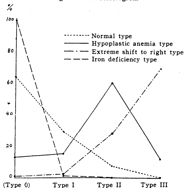
Fig. 3. Sideroblastogram
