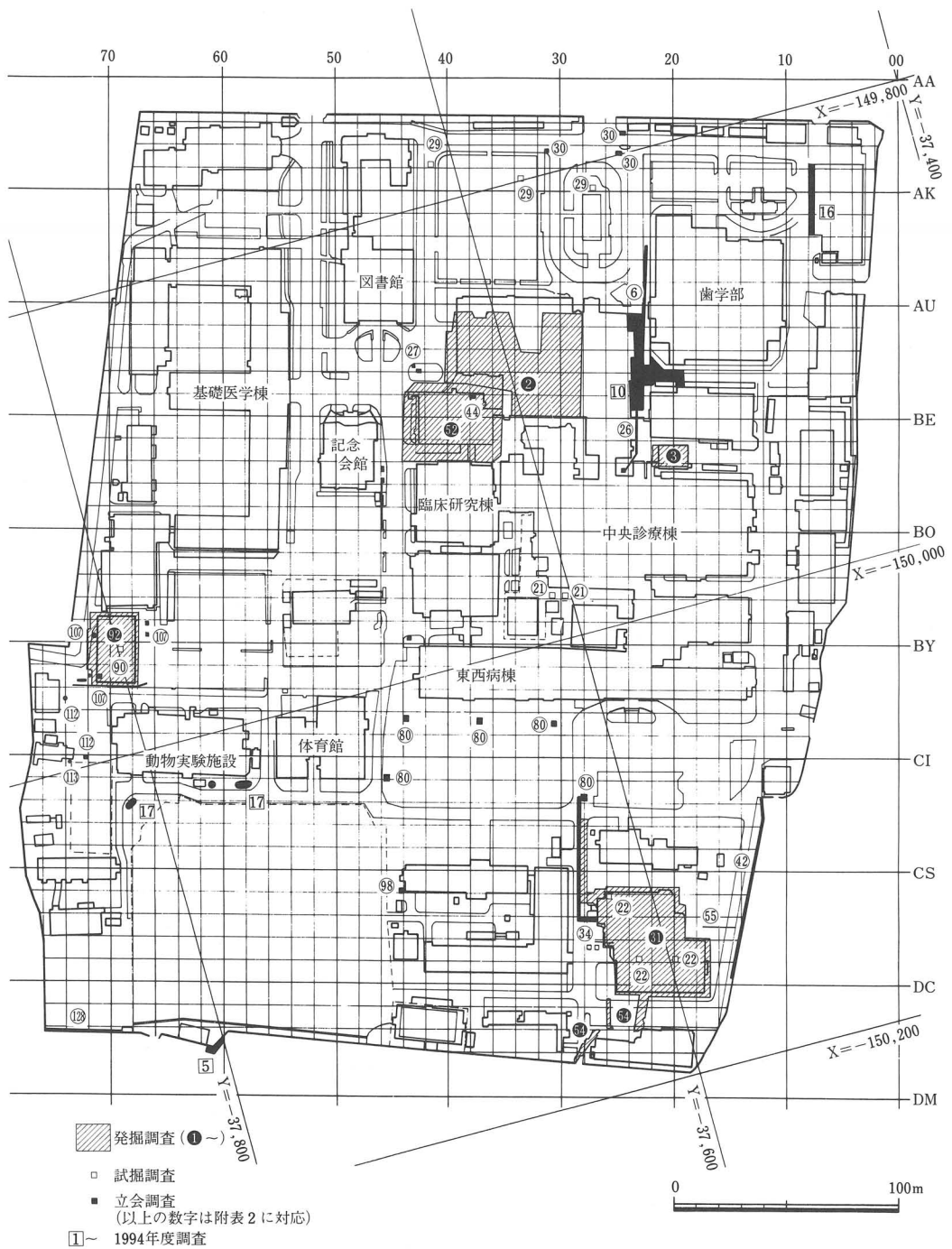
図15 1994年度までの調査地点(2) 鹿田地区 (縮尺1/3,000)
