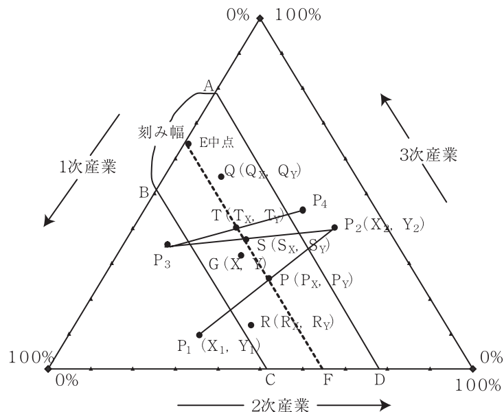
図3 産業構造三角形ダイアグラム
