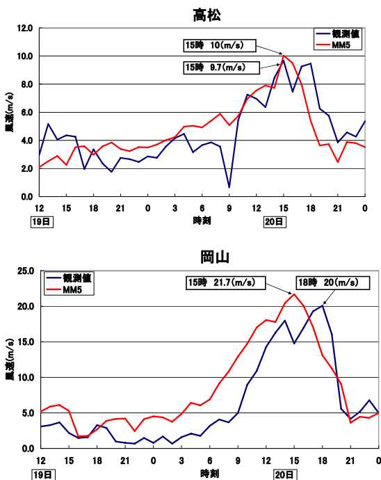
図 18 台風 23 号における高松・岡山での MM5 と観測値の風速の比較
